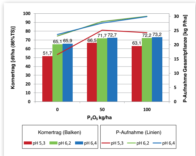
Abbildung 4: Einfluss des pH-Werts des Bodens auf die P-Verfügbarkeit (Quelle: Tucher, 2016)
