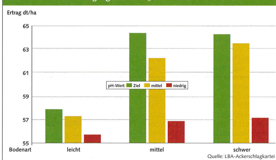
Abb. 1: Ertragsleistung von Wintergerste in Abhängigkeit von Bodenart und Kalkversorgung (Probenzahl gesamt: 8.414)
